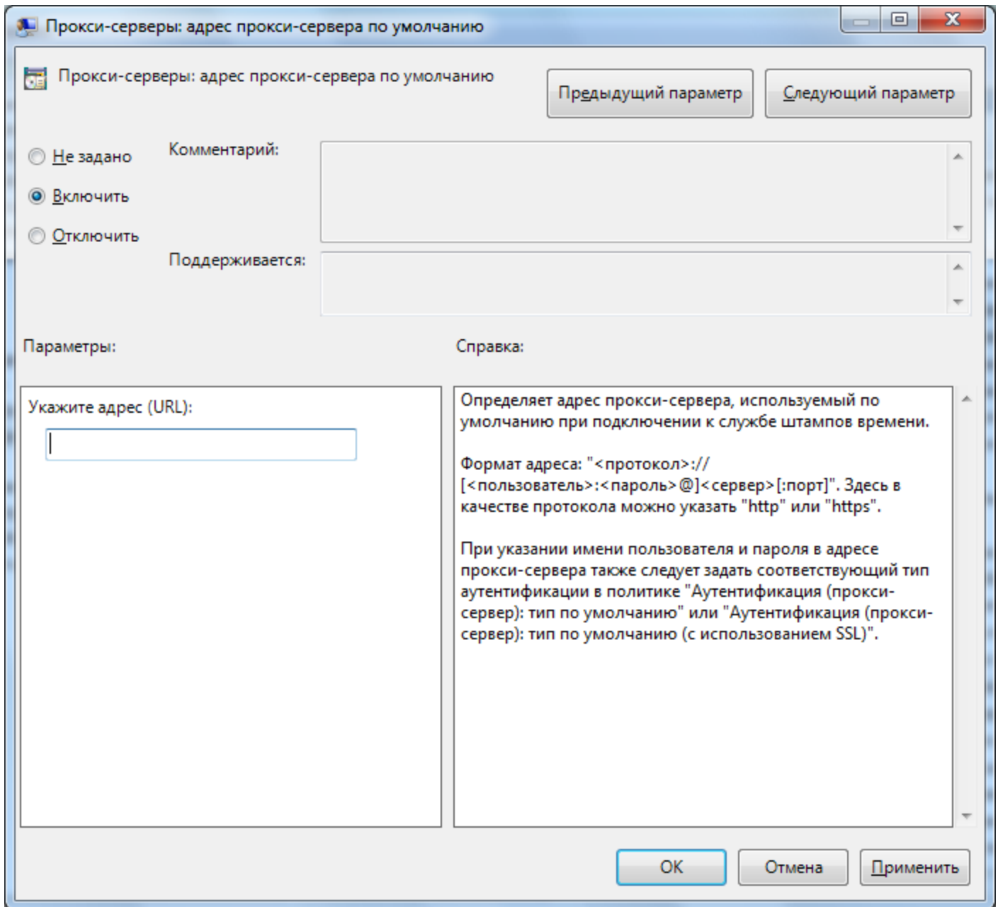
Рис.3. Настройка адреса прокси-сервера
